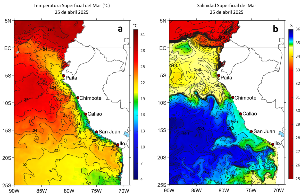
Figura 2. a) Temperatura superficial del mar (°C) y b) Salinidad superficial del mar para el 25 de abril del 2025. Datos: OSTIA-UKMO-L4-GLOB-v2.0 (UK Met Office, 2012; Donlon et al, 2012) y del GLOBAL_ANALYSISFORECAST_PHY_001_024 (Lellouche, J. M. et al, 2013), respectivamente.
