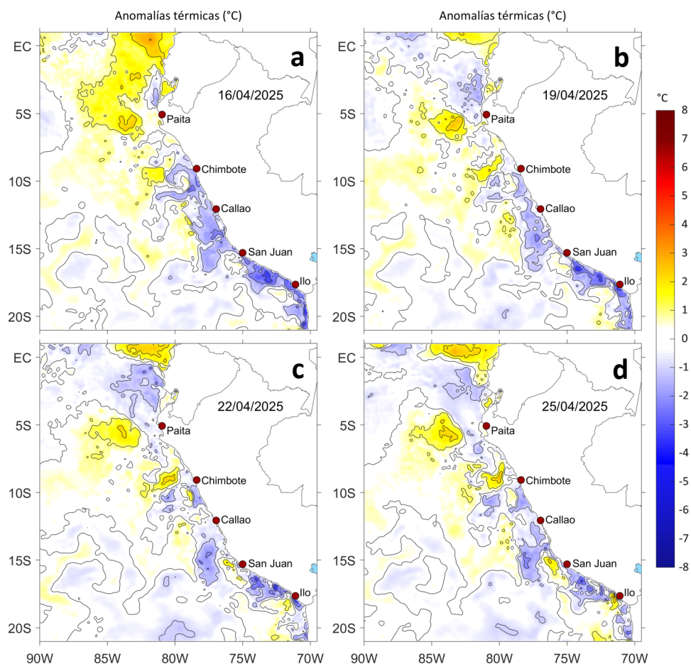
Figura 3. Anomalías de la temperatura superficial del mar (°C) para el a) 16, b) 19, c) 22 y d) 25 de abril del 2025. Las anomalías se calcularon respecto de la climatología para el periodo 1991-2020. Datos: OSTIA-UKMO-L4-GLOB-v2.0 (UK Met Office, 2012; Donlon et al, 2012).
